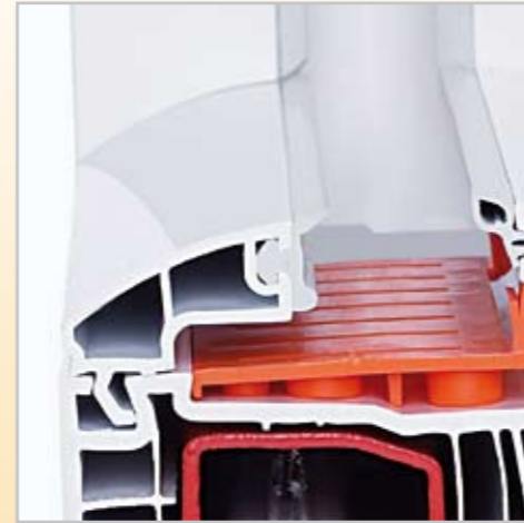
Bogenglasleiste
